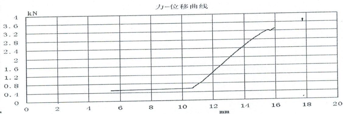
单股钢丝拉断测试 第三次
