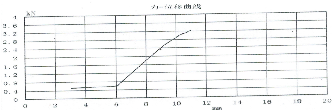
单股钢丝拉断测试 第二次
