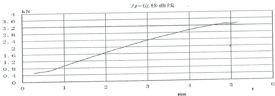
单股钢丝拉断测试 第一次
